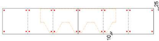
Рис. 16. Схема крепления коньково-карнизной черепицы Döcke PIE на карнизе.
