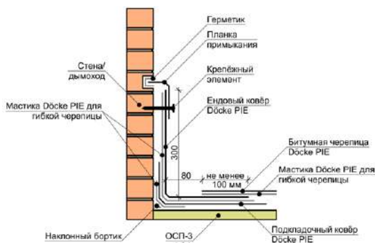
Рис. 29. Примыкание ската крыши к выступающим над ней конструкциям под углом более 90°.
