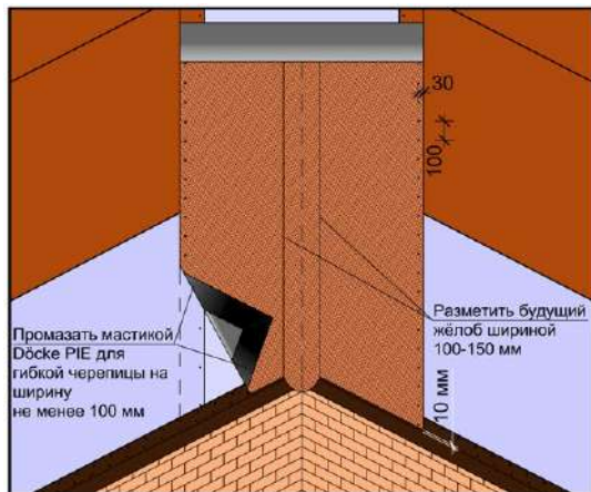
Рис. 13. Монтаж ендового ковра.
